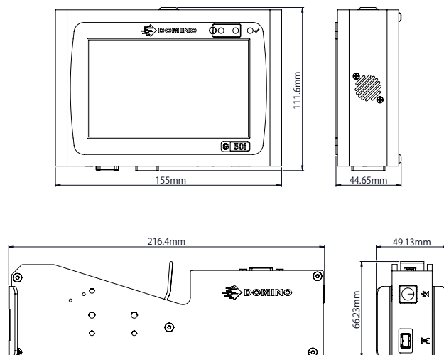
寸法図
