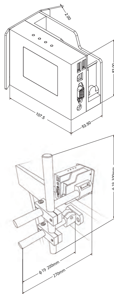
寸法図
